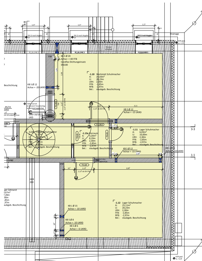
Lagerfläche
