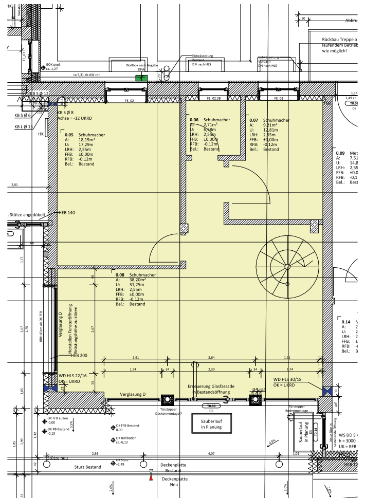
Gewerbefläche
