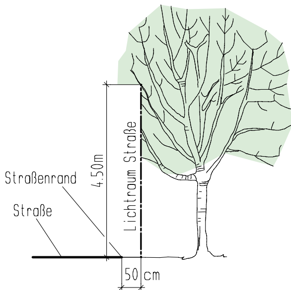
Freizuhaltender Lichtraum neben Straßen
