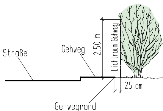
Freizuhaltender Lichtraum neben Gehwegen
