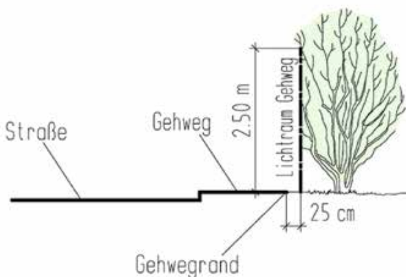
Freizuhaltender Lichtraum neben Gehwegen
