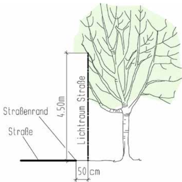
Freizuhaltender Lichtraum neben Straßen
